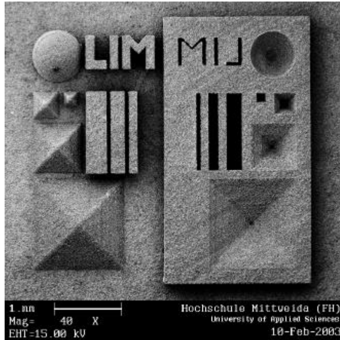
Hochaufgelöste 3D Sinterstruktur aus Wolfram
